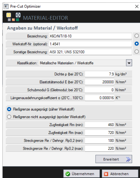
Bild 3-10: Material-Editor – Standard-Ansicht
